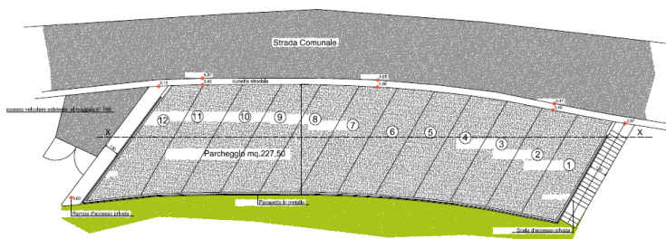
Planimetria del nuovo parcheggio pubblico su via San Fedele di prossima realizzazione antistante il parcheggio esistente al servizio del centro storico
